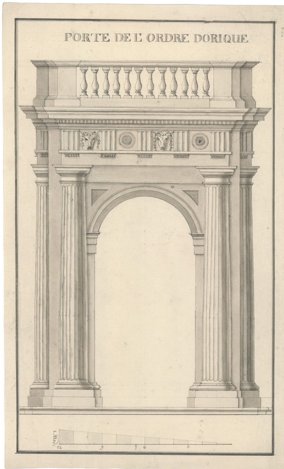
Tekening uit de 'Plans de l'architecture civile et militaire faits et lavez par Monsieur G. de Spaen'
